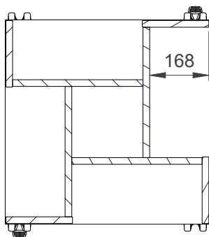
A-A ( 1 : 15 )
